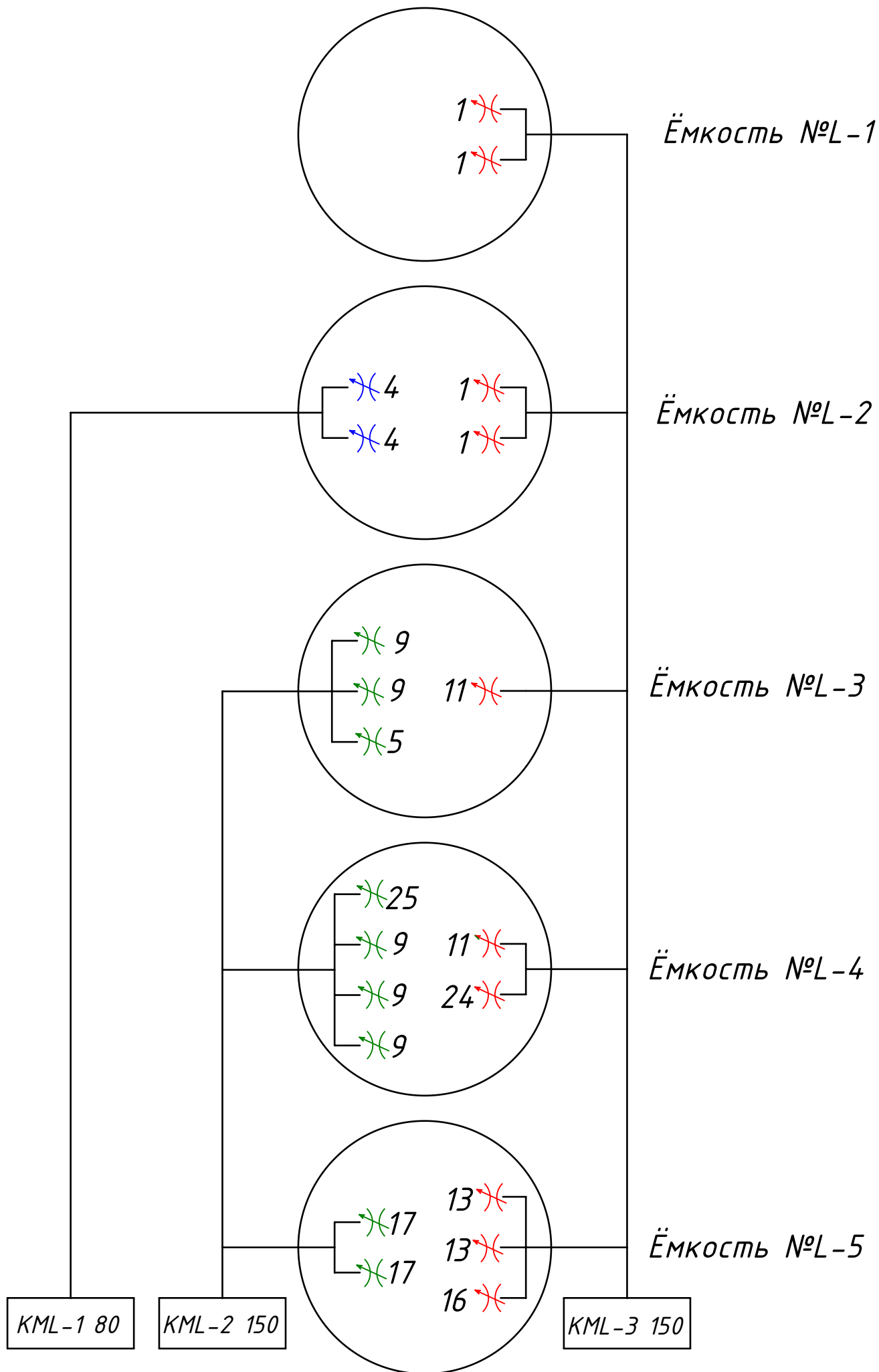
Схема потребления воздуха Коло Илта 200 линии №№1-2 (L-номер линии)
